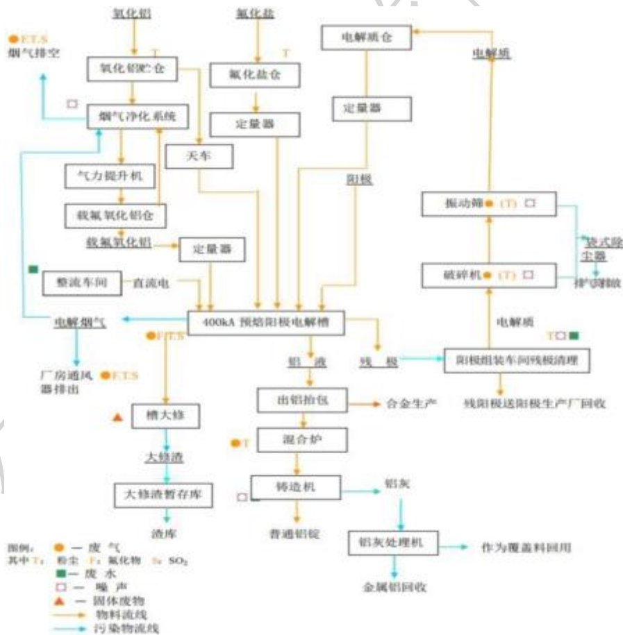
图 2 排放单位电解工艺流程图
